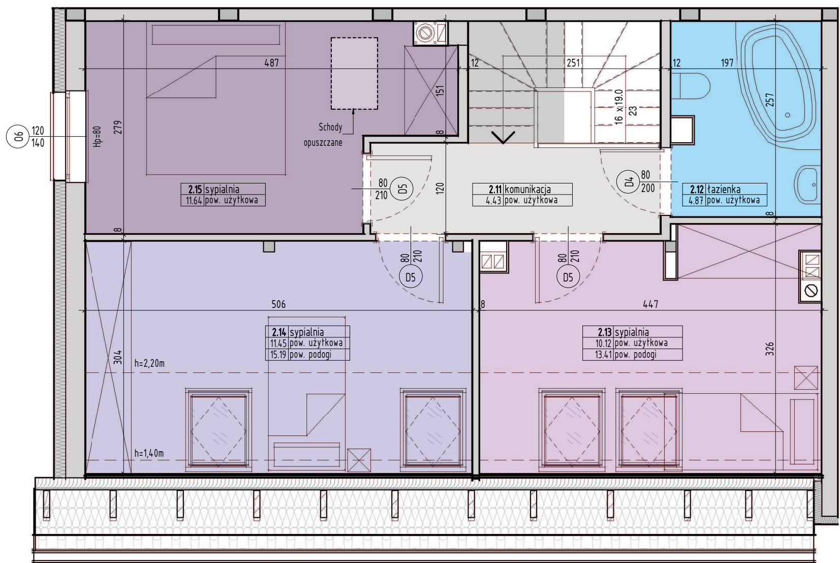
RZUT PODDASZA
