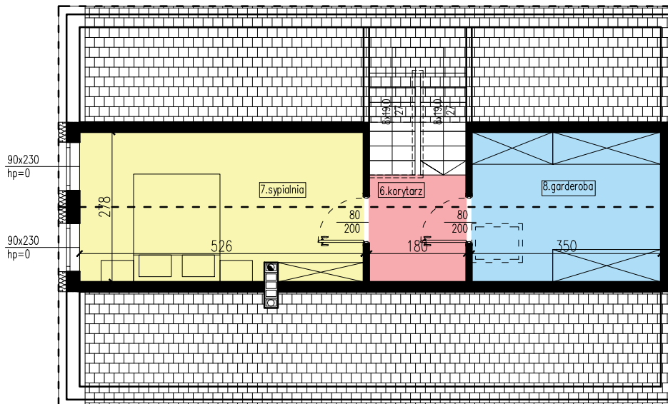
RZUT PODDASZA
