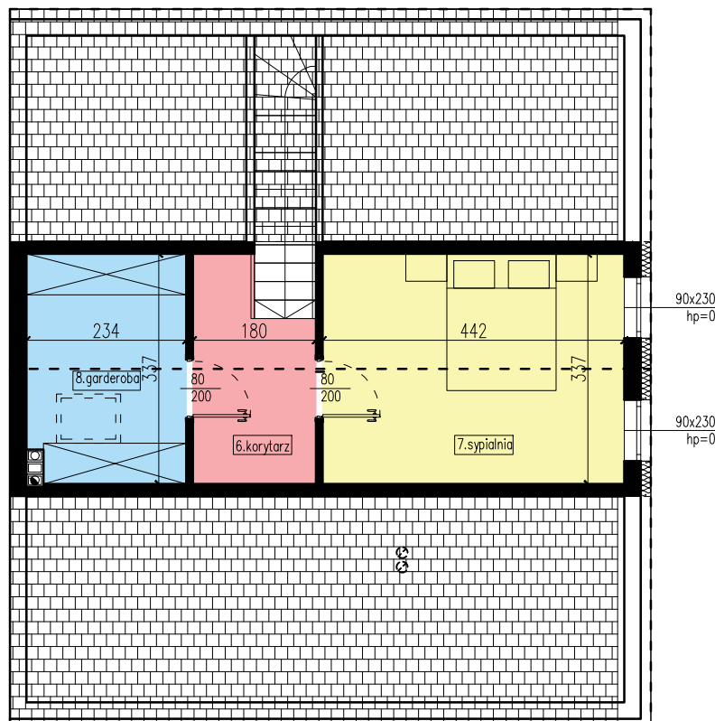
RZUT PODDASZA
