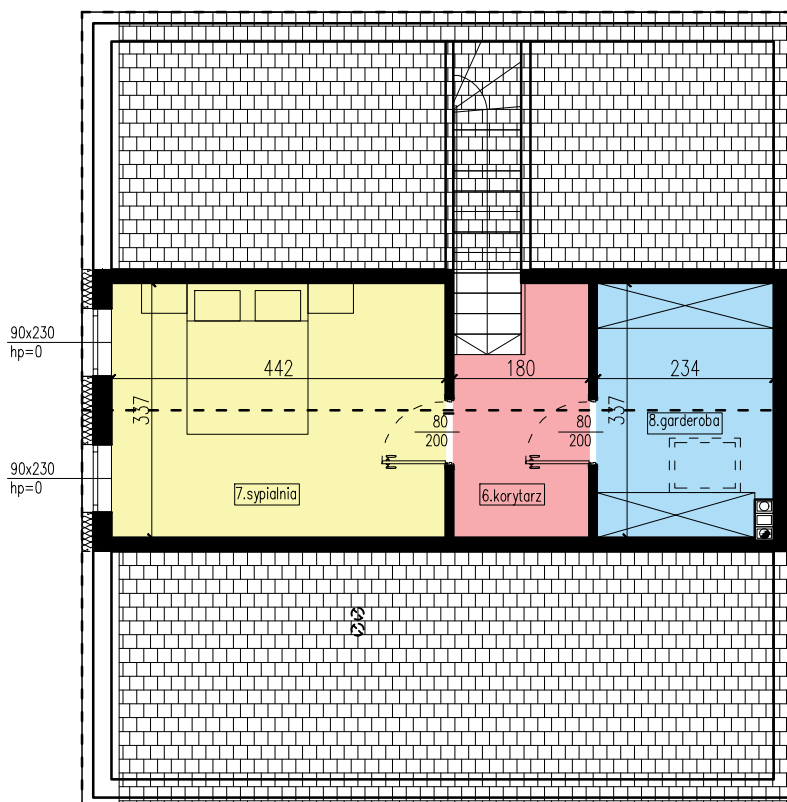
RZUT PODDASZA
