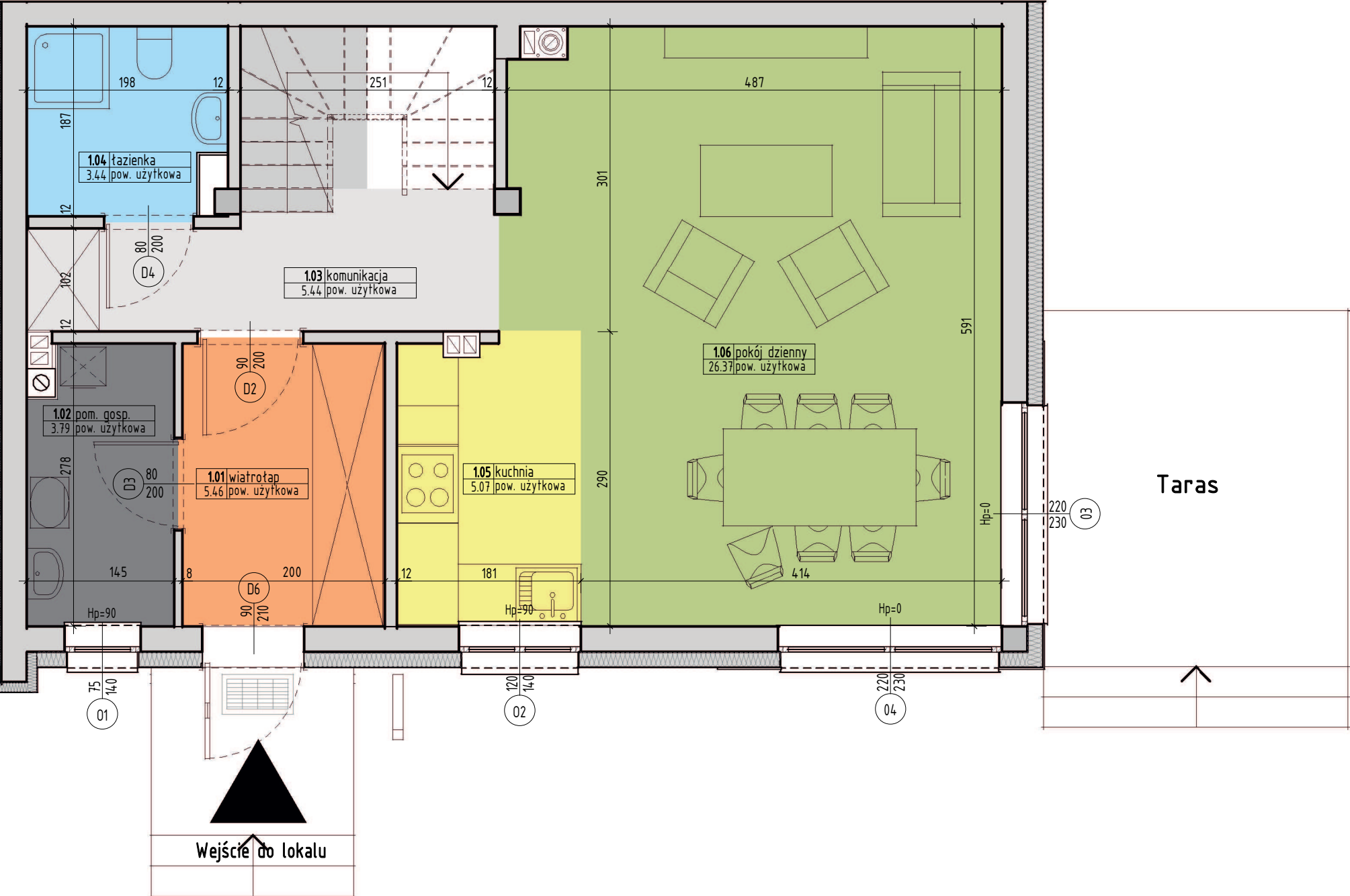
RZUT PARTERU
