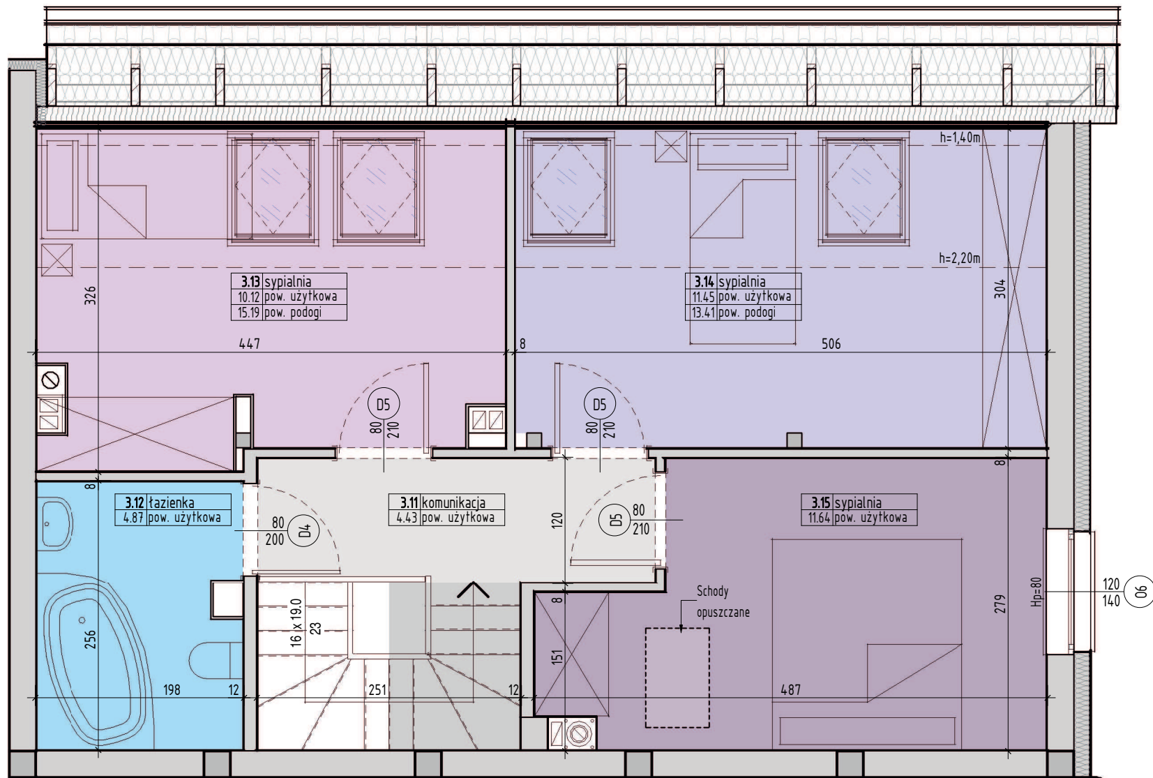
RZUT PODDASZA
