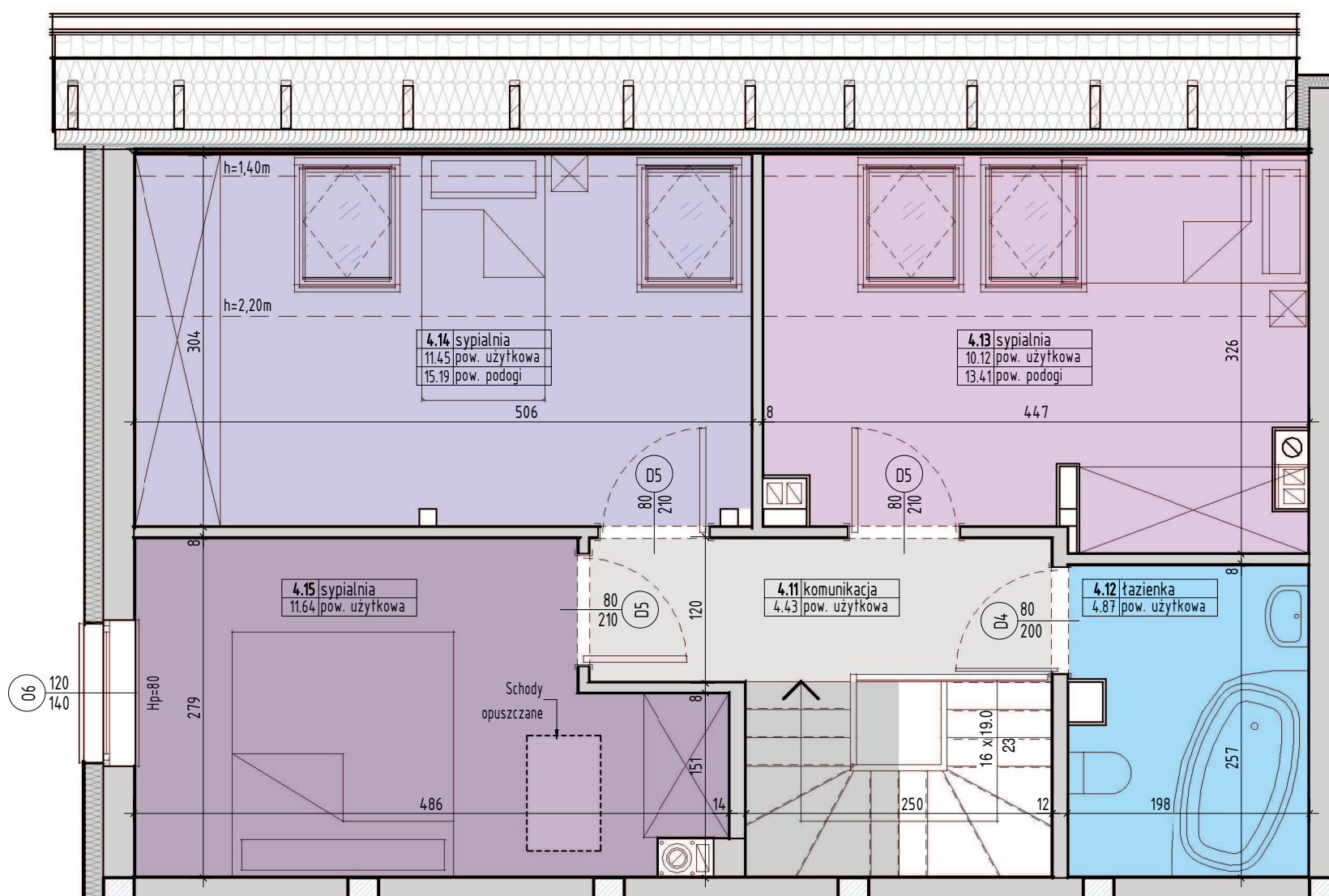
RZUT PODDASZA
