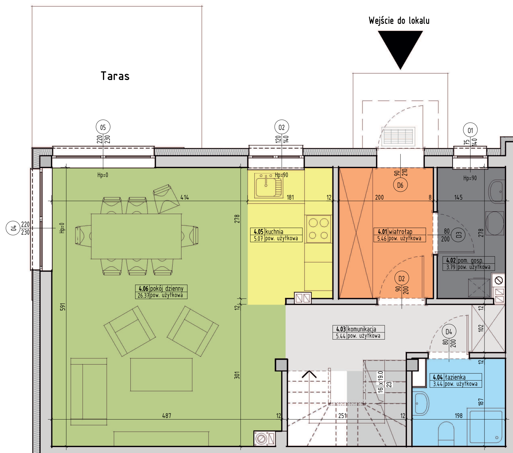
RZUT PARTERU
